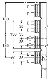
E4 Вид А
