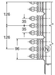
E6/f Вид А
