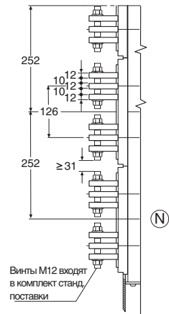
E6/f Вид А
