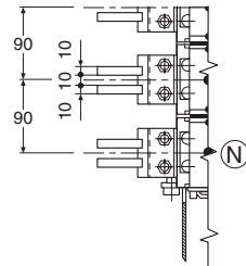
E2 Вид А
