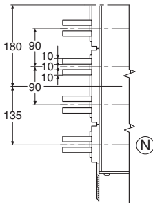
E4 Вид А
