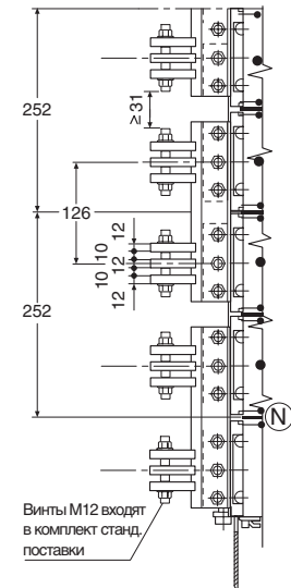
E6/f Вид А
