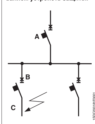
Электрическая схема с селективным согласованием устройств защиты.
