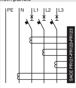
Трехполюсные автомат. выключатели с внешней нейтралью
