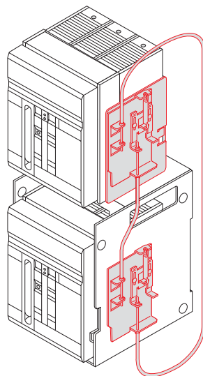
вертикальная взаимная блокировка
