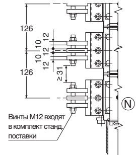
E3 Вид А
