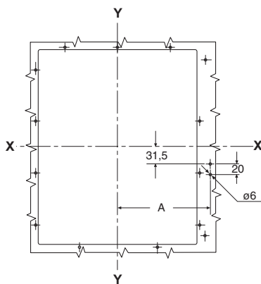
A эполюсн. 4-полюсн.
