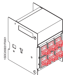
Плоские выводы
