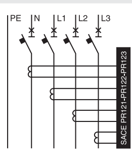
Четырехполюсные автомат. выключатели
