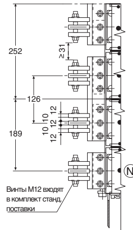
E6 Вид А
